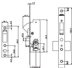
6917-Z-IP Acabamentos: IP/IEP/IEB Broca 17 mm
