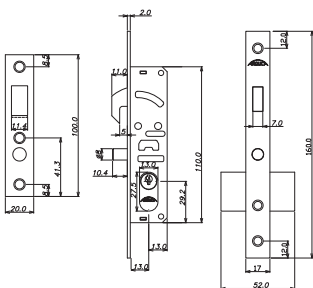
6915-Z-IP Acabamentos: IP/IEP/IEB Broca 13 mm
